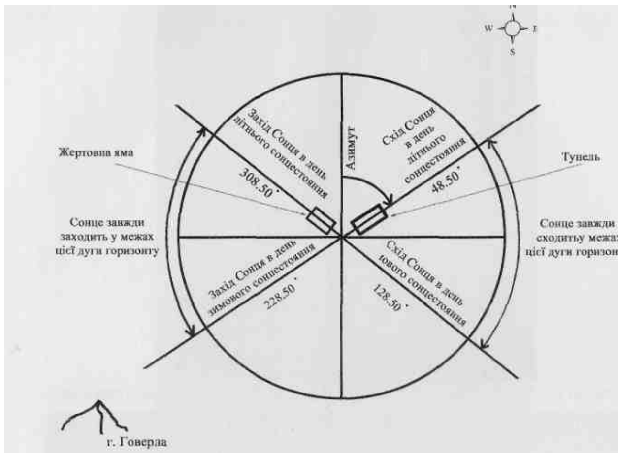
Малюнок 5. Орієнтовні азимути для точок сходу і заходу Сонця на широті Лисини Космацької (за Т. Маланюком і Р. Сливкою)
